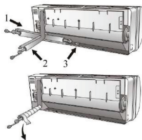
Распрямление соединительной трубы
