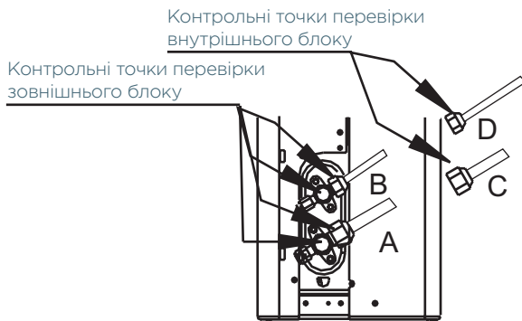
A: Запірний клапан низького тиску B: Запірний клапан високого тиску C і D: Конусні гайки внутрішнього блоку
