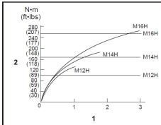
Правильний момент затягування для високоміцного болта.
