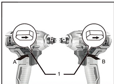
1. Кнопка перемикачя реверса
